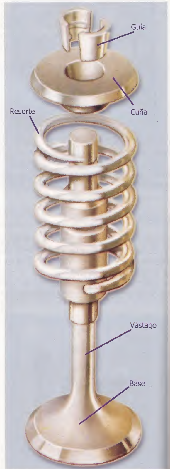
Válvula completa de motor de cuatro tiempos
